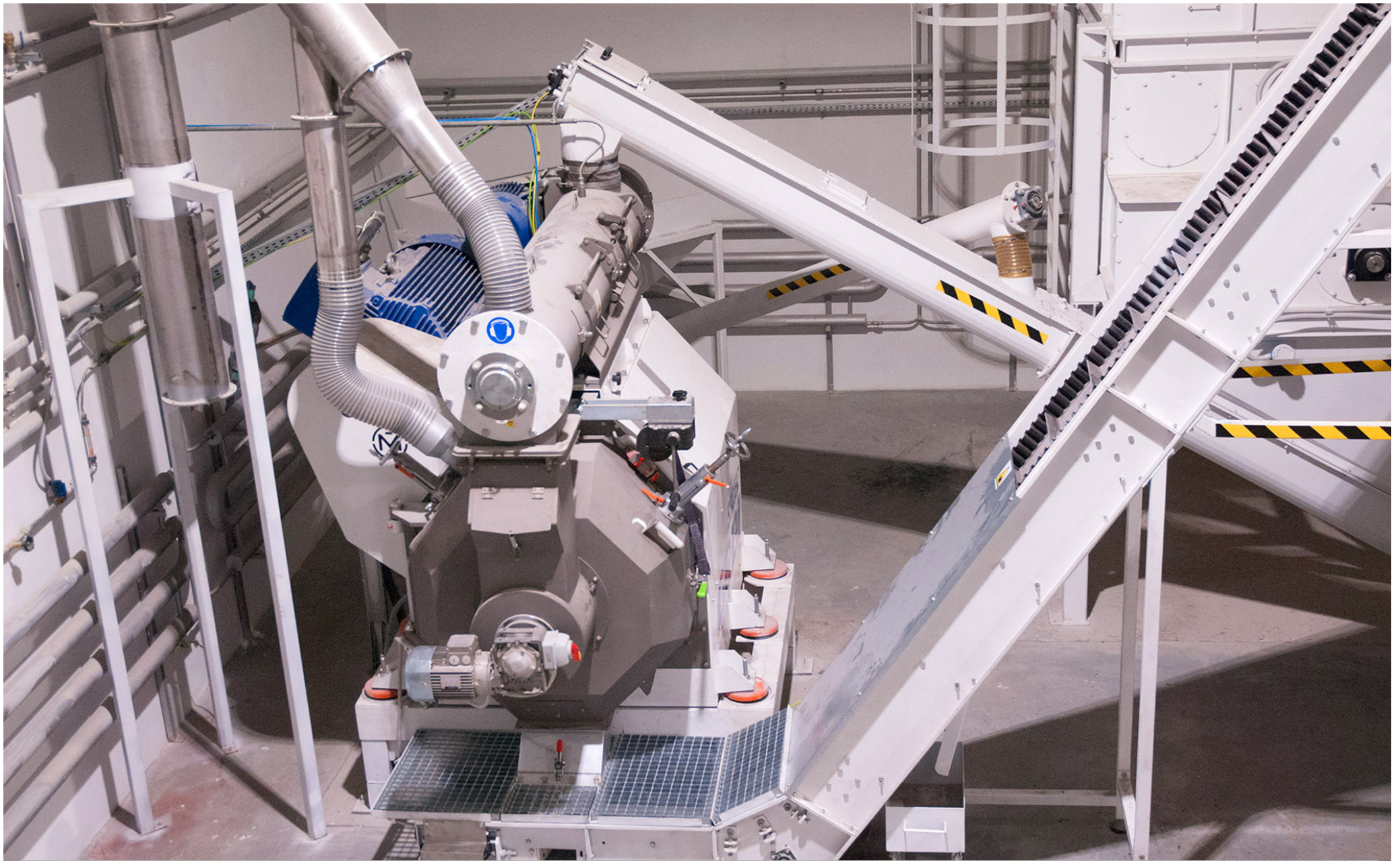
GRANULATOR GRB1 550.132 NA KONSTRUKCJI Z PRZENOŚNIKIEM TAŚMOWYM (ŁAMANY 2X)
