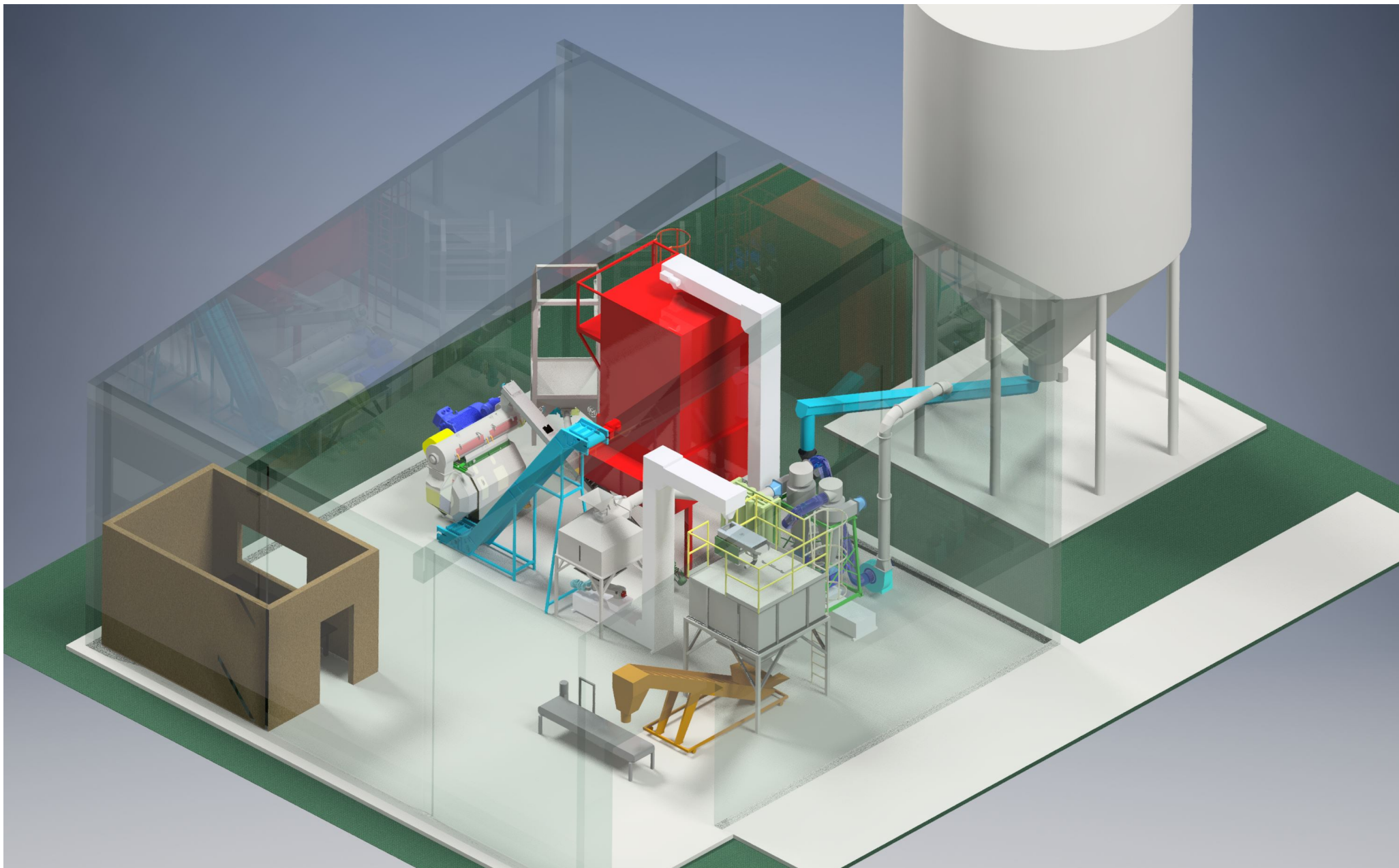
PNEUMATYCZNY TRANSPORT SUROWCA Z MŁYNA DO ZBIORNIKA BUFOROWEGO GRANULATORA
